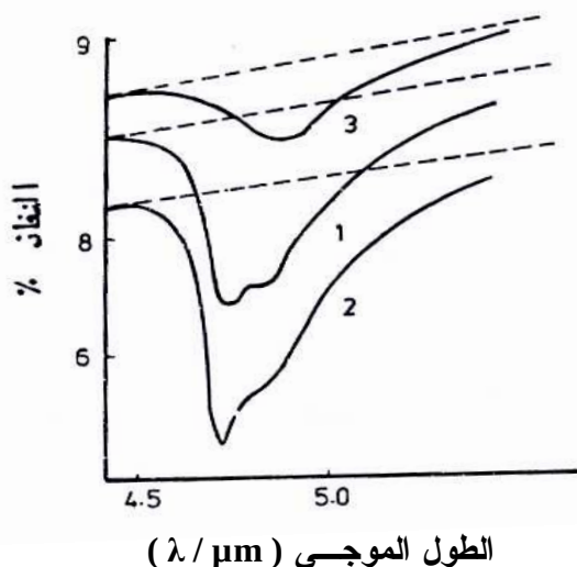
طيف تحت الحمراء للهيدروجين الممتز على البلاتين
