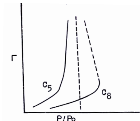
أيزوثيرم الامتزاز للبنتان والاوكتان في ١٥° مئوية
